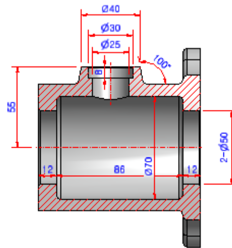
'단면 A-A'
