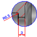
'상세부 E (2:1)'
