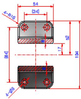
'단면부 A-A'
