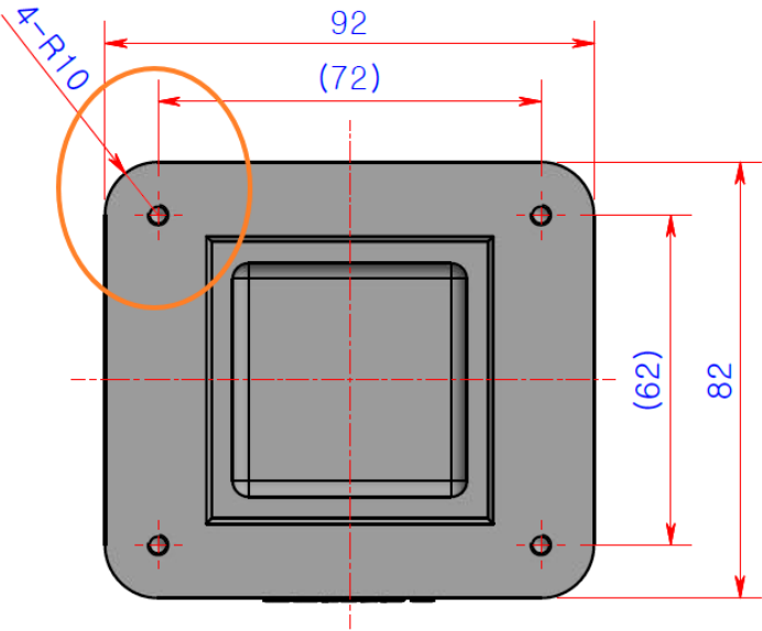
치수기입 표시
