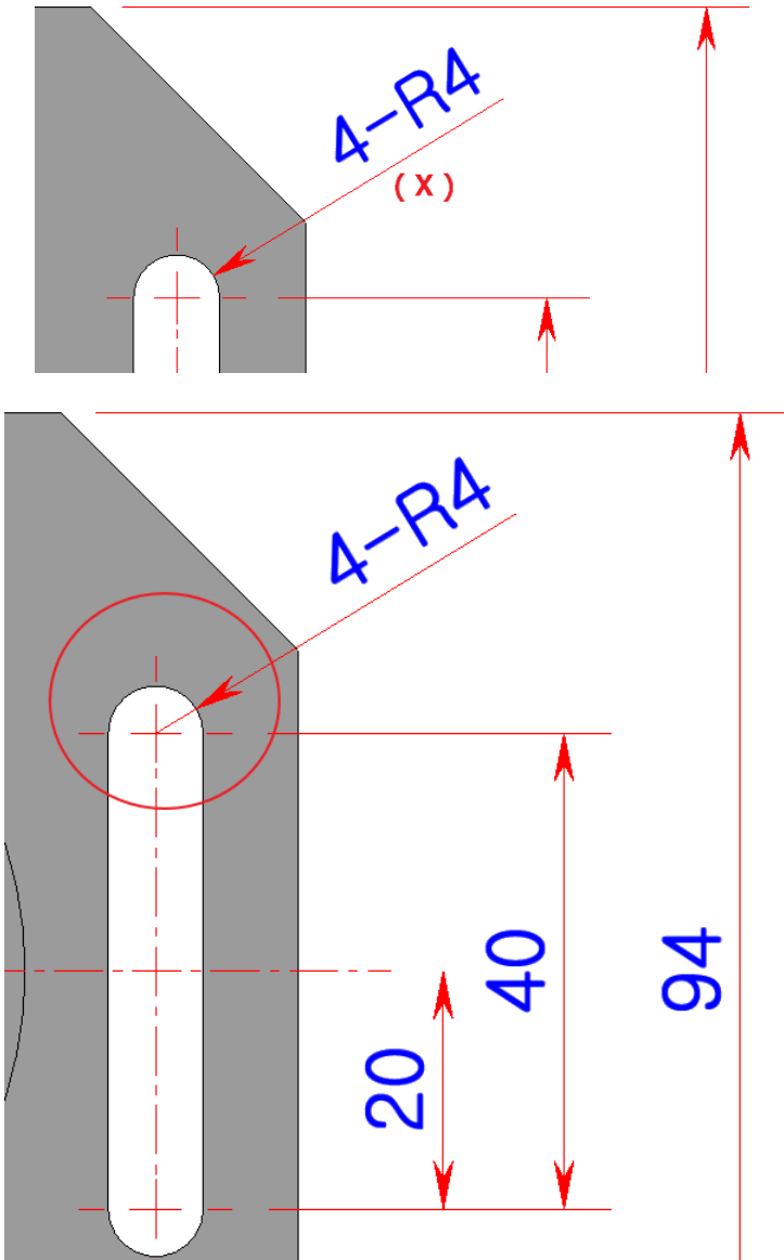
치수기입 (-2)
