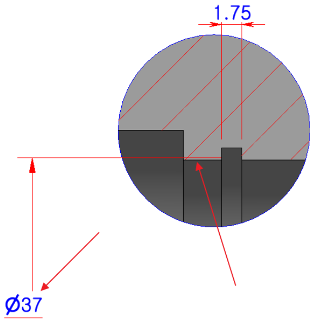
치수기입 (-2)
