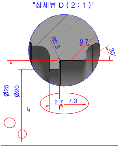
치수기입 (-4)
