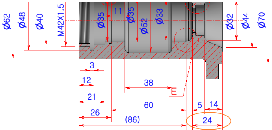
괄호 치수기입 (-2)
