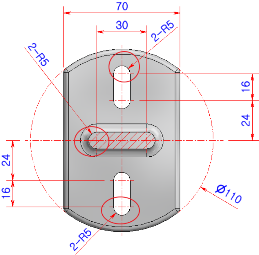
" 단면뷰 A-A "
