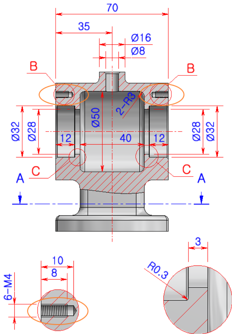
" 상세뷰 B (1:1) "
