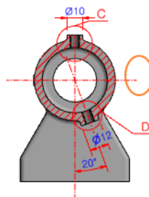
단면뷰 A-A
