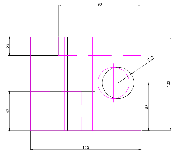
RIGHT SCALE: 1/2
