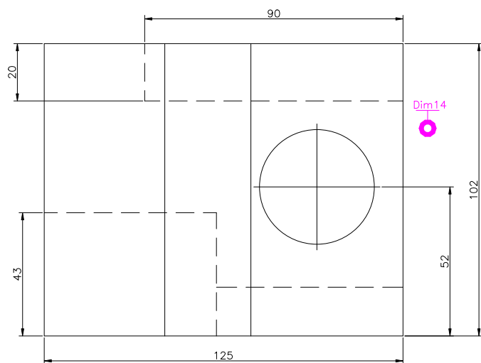
FROLT SCALE 1/2
