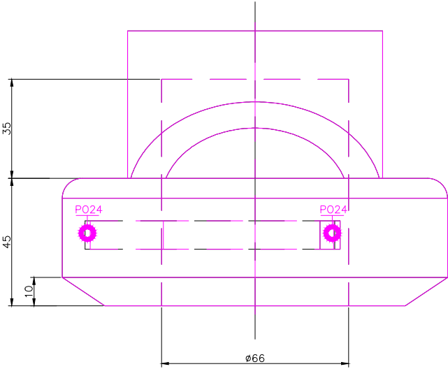
RIGHT SCLAE 1/2
