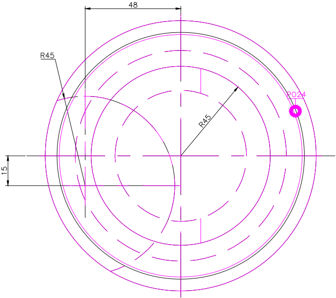
TOP SCLAE 1/2
