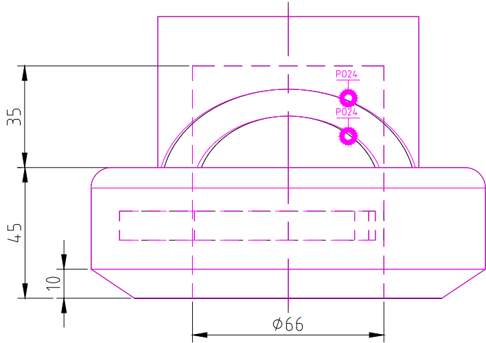
RIGHT SCLAE 1/2
