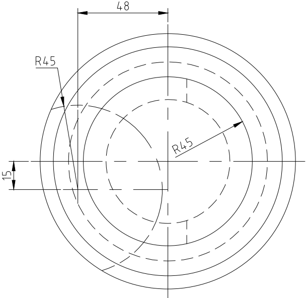
TOP SCLAE 1/2
