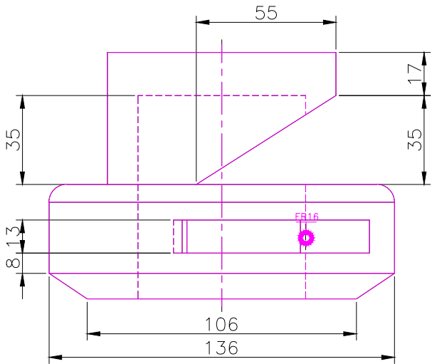
RIGHT SACLE 1/2
