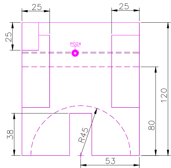
RIGHT SCLAE 1/2
