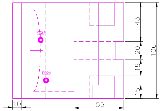
TOP SCLAE 1/2
