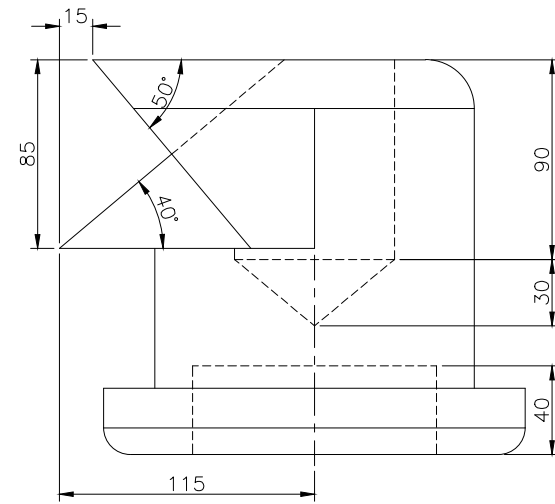
RIGHT SCLAE 1/3
