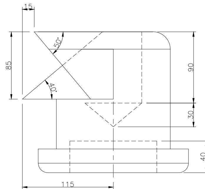
RIGHT SCALE : 1/3
