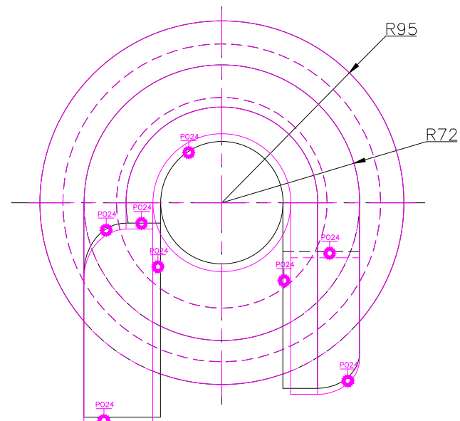
TOP SCALE : 1/3
