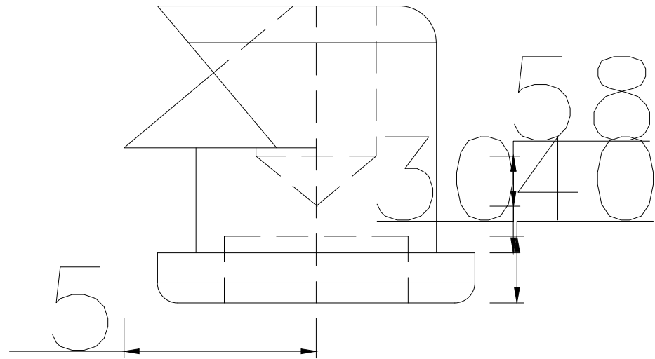
right scale : 1/2
