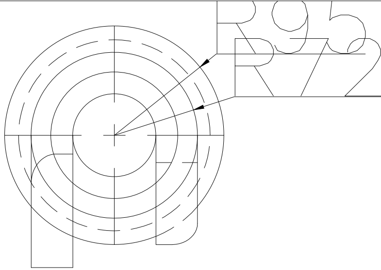
top scale : 1/2
