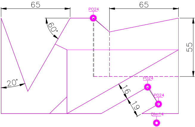
TOP SACLE
