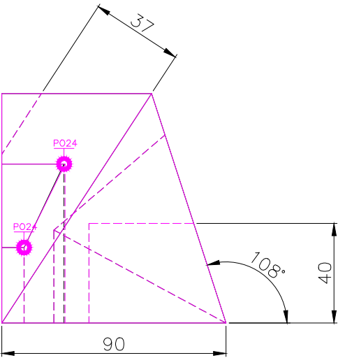
RIGHT SACLE
