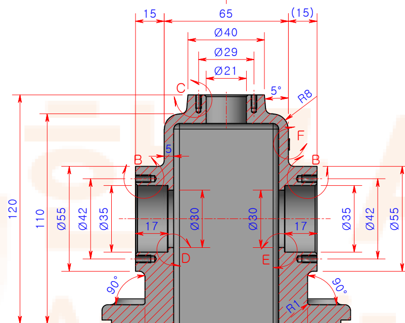
"단면뷰 A-A"
