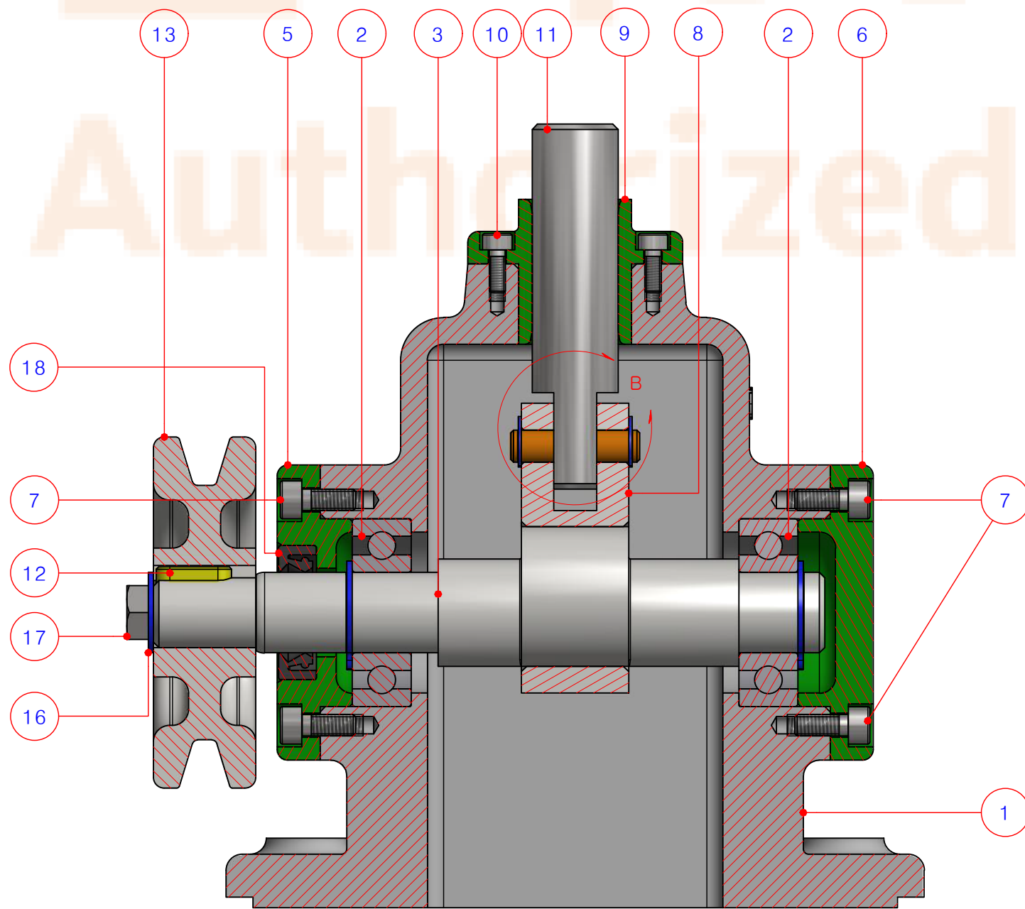
"단면뷰 A-A"
