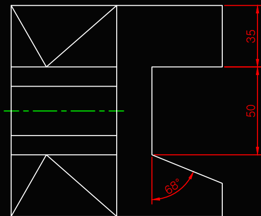
TOP
