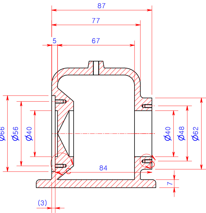
'단면뷰A-A'
